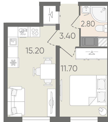
1-комнатная квартира с европланировкой
